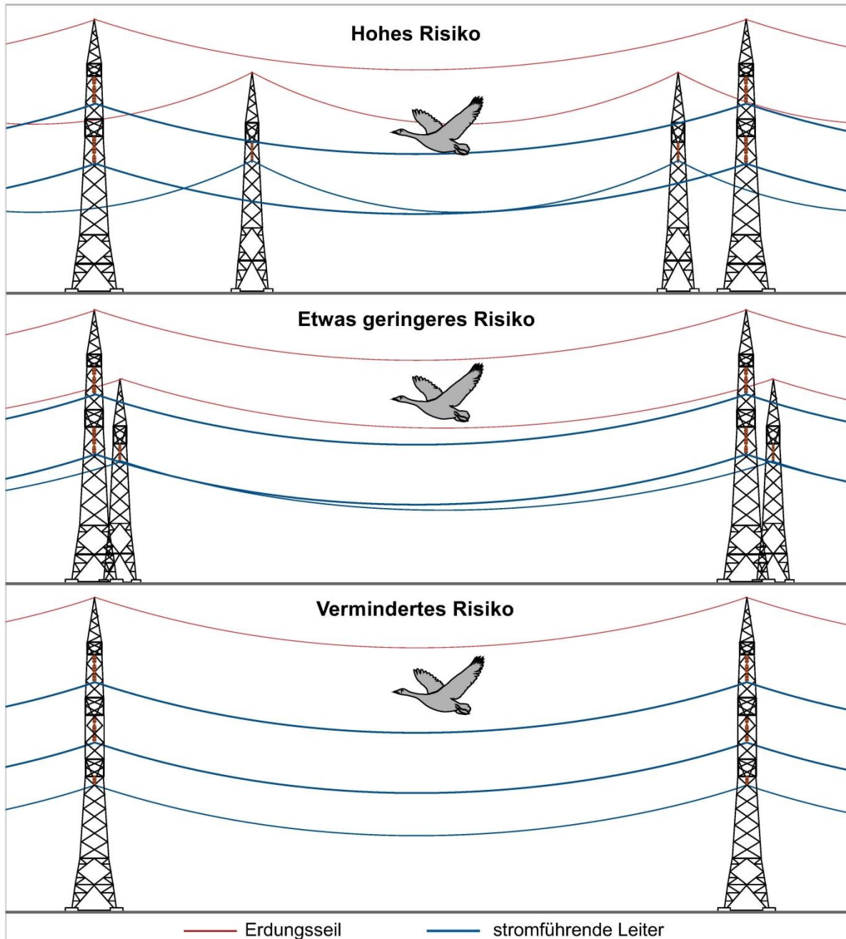
Abb. 21: Mögliche Reduktion des Kollisionsrisikos von Freileitungen durch Synchronisation mit oder Mitnahme von weiteren Leitungen (nach THOMPSON 1978 bzw. APLIC 2012).
