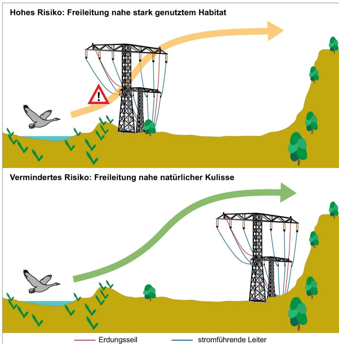
Abb. 19: Berücksichtigung topografischer Strukturen bei der Trassierung (nach THOMPSON 1978 bzw. APLIC 2012).
