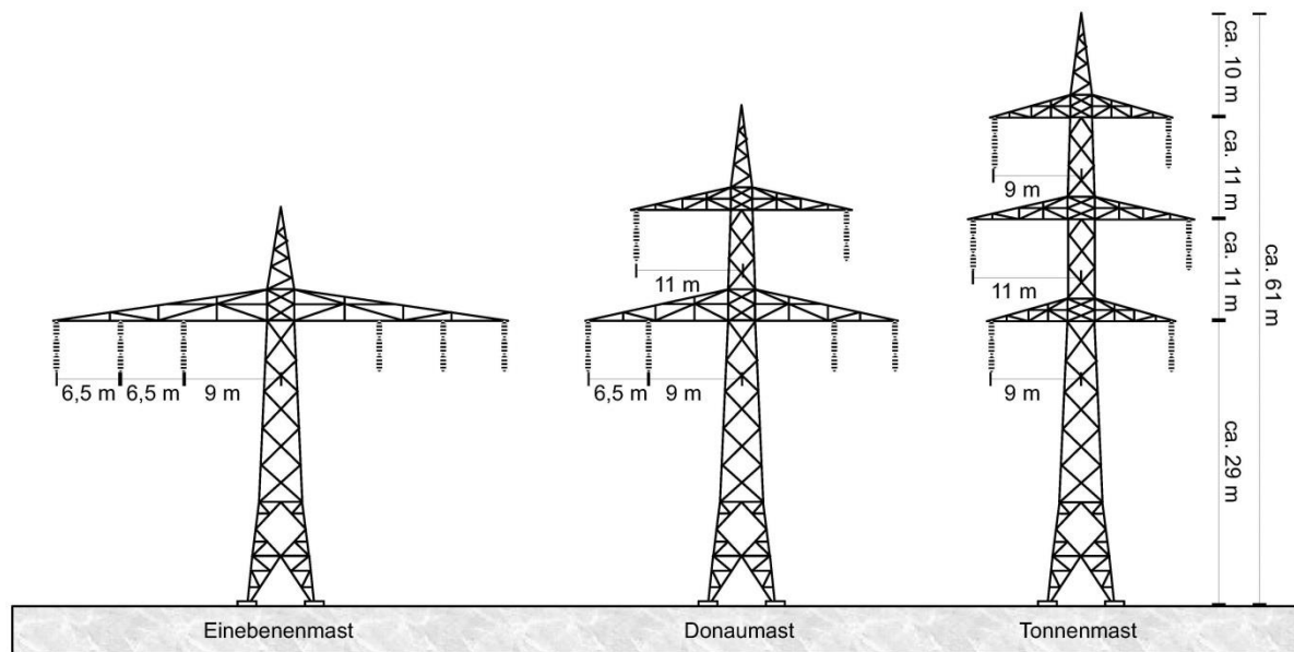
Abb. 13: Schematische Darstellung von Eiebenen-, Donau- und Tonnenmast (nach HOFMANN et al. 2012: 9).
