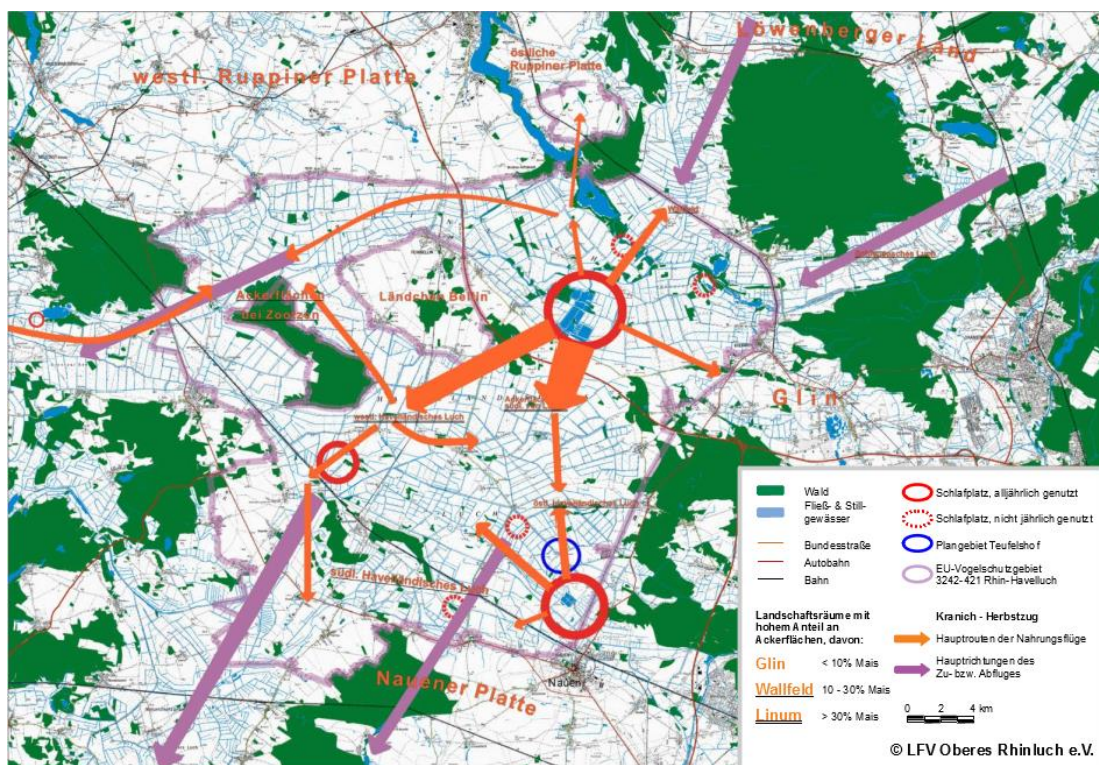
Abb. 12: Hauptflugrouten und Schlafplätze der Kraniche im Rhin-Havelluch während der Herbstzeit, rote Kreise = alljährlich genutzte Schlafplätze, Pfeile = Hauptflugrouten (LANDSCHAFTSFÖRDERVEREIN OBERES RHINLUCH 2015).
