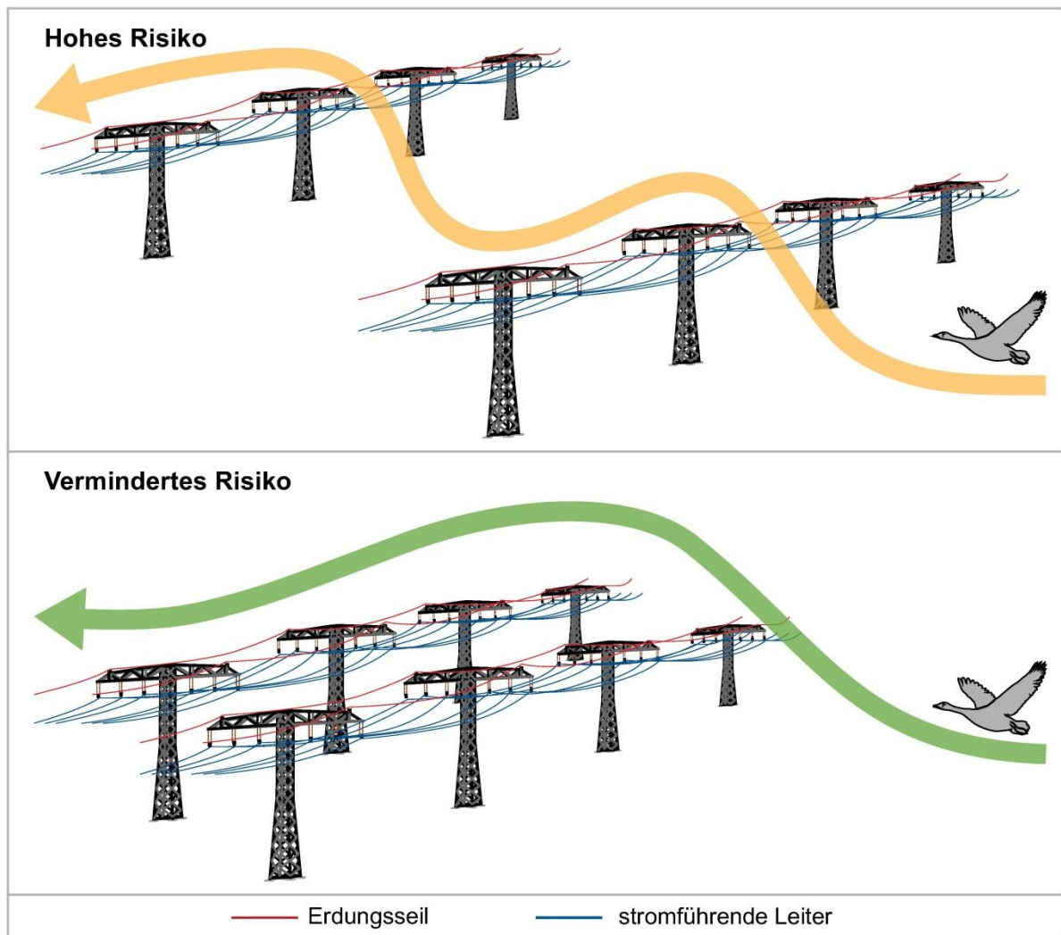
Abb. 20: Kollisionsrisiken an ungebündelten und gebündelten Freileitungen (nach THOMPSON 1978 bzw. APLIC 2012).
