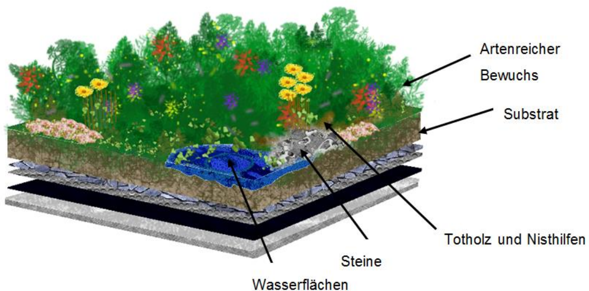
Abbildung 6: Dachaufbau eines die Biodiversität fördernden Daches mit strukturreicher Ausstattung folgender Habitatelemente: Totholz, Nisthilfen, Wasserflächen, Steinen und Anhügelungen. Grafik: Dr. Sebastian Schmauck, BfN
