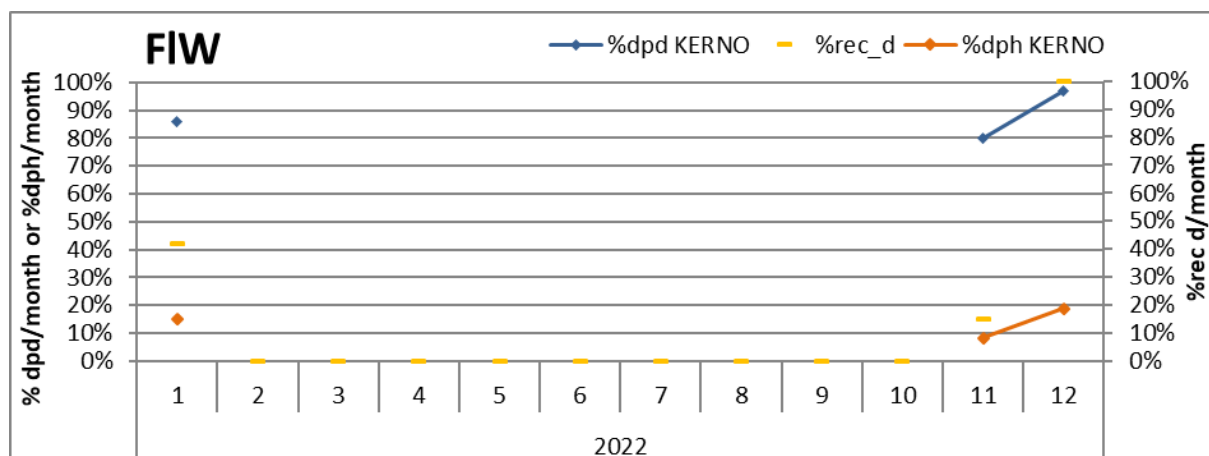
Abbildung 2: Schweinswalpositive Tage (dpd, blaue Linien) oder Stunden (dph, orange Linien) pro Monat in % sowie Anteil an observierten Tagen pro Monat in % (gelbe Striche) an der Station FIW in 2022.
